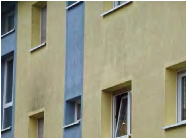
Bild 11–14: Die hellen Flecken auf den beiden linken Fotos stammen von Metalldübeln, die wärmer sind als die Dämmung
